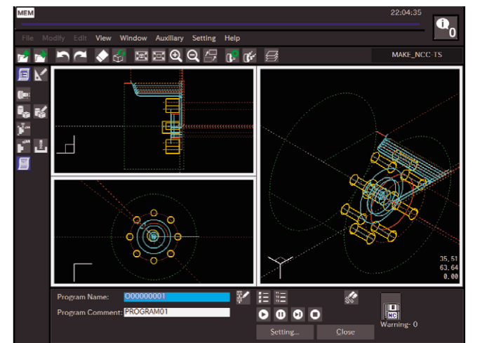
车床用对话画面
